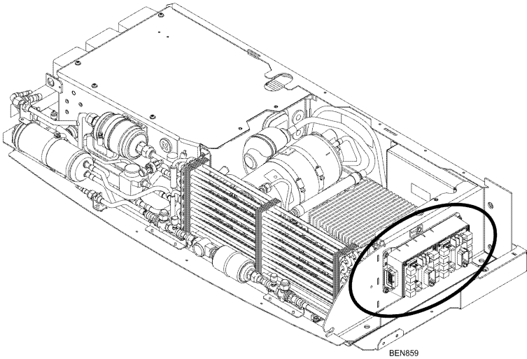
Ilustración 9. Ubicación de los fusibles (cubierta del condensador retirada)
