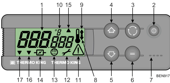
Ilustración 7. Pantalla, teclas y símbolos del panel de control en cabina (HMI)
